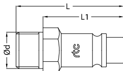
Plug / Nippel
