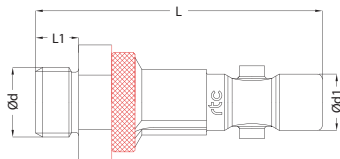
Plug / Nippel
