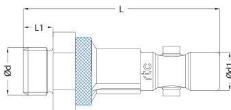
Plug / Nippel
