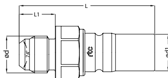
Plugs / Nippel
