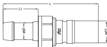
Plugs / Nippel
