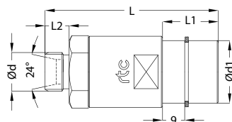
Plug / Nippel
