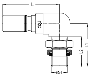
Plug / Nippel
