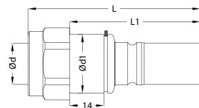
Plug / Nippel
