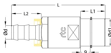
Plug / Nippel
