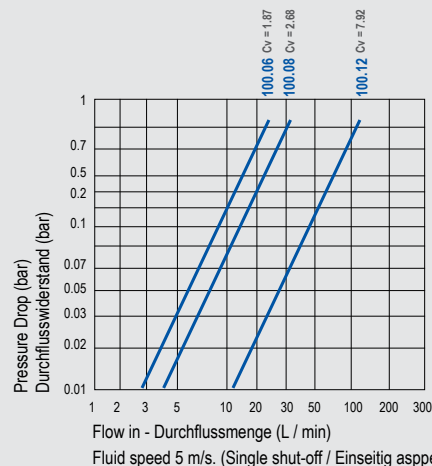
Flow Rate vs Pressure Drop Graph / Durchflussrate vs Druckabfall
