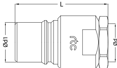
Plug / Nippel
