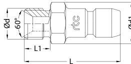
Plug / Nippel
