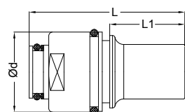
Plug / Nippel
