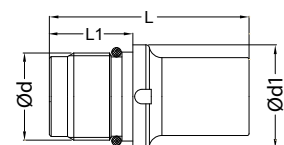
Plug / Nippel
