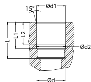
Plug / Nippel
