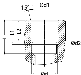
Plug / Nippel
