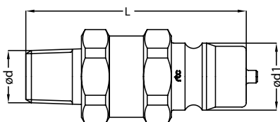
UNF Male thread plug with 37° sealing cone / Nippel mit UNF Aussengewinde 37° Dichtkonus
