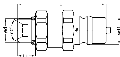
Male conical thread plug / Nippel mit Aussengewinde konisch
