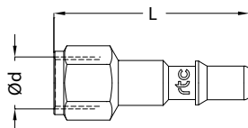
Female thread plug / Nippel mit Innengewinde
