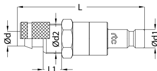
Plugs / Nippel
