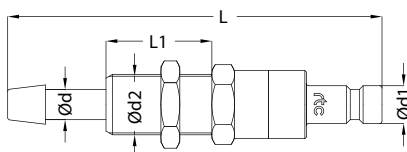
Plugs / Nippel
