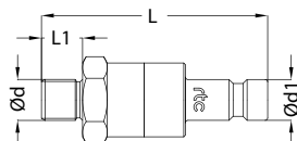
Plugs / Nippel
