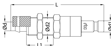
Plugs / Nippel
