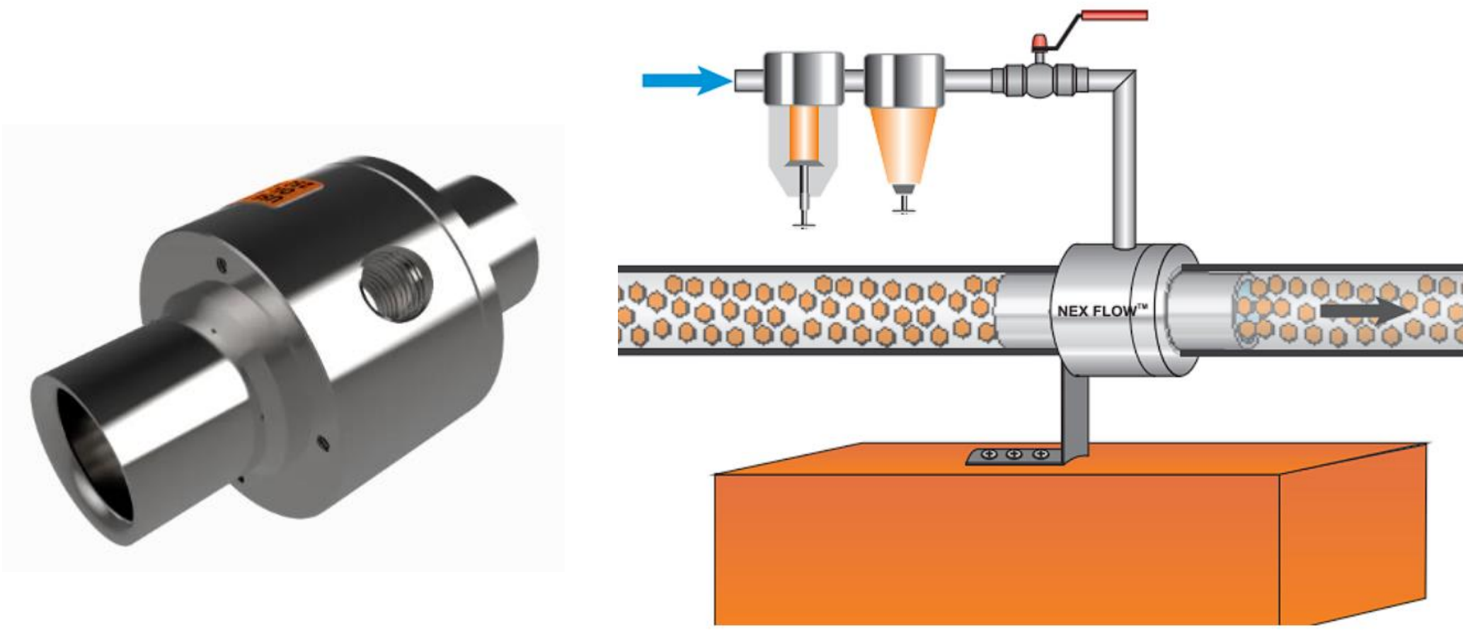
Pnömatik Konveyörler
